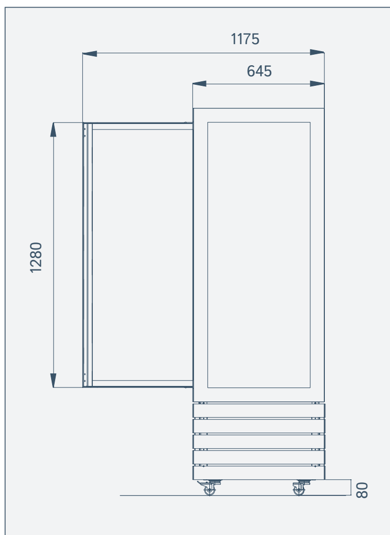
VISTA LATERALE
