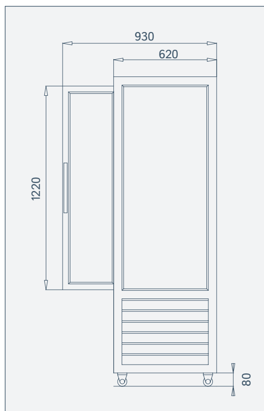
VISTA LATERALE
