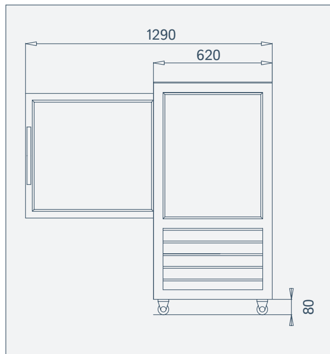
VISTA LATERALE
