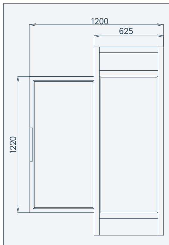
VISTA LATERALE Side view / Seitenansicht / Vue latérale
