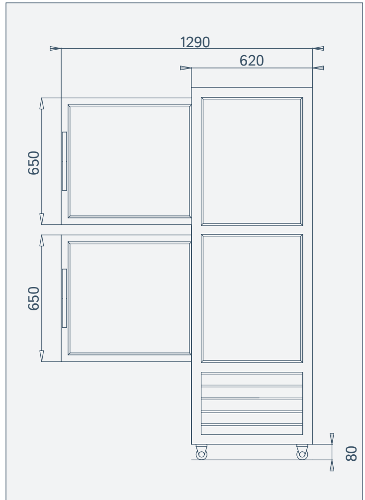
VISTA LATERALE
